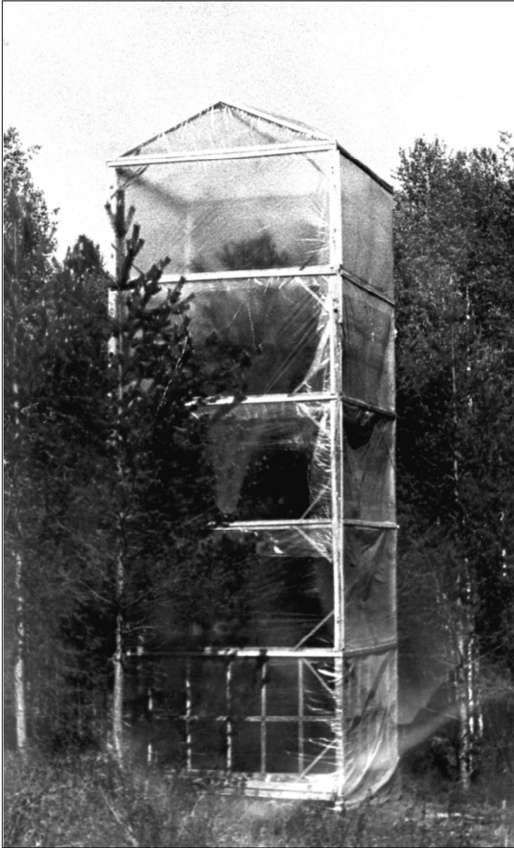
Сборная пленочная камера для подкормки сосны \text{CO}_2 . Конструкция к.б.н., с.н.с. П.В. Тихова. Карелия, 1980 г.
